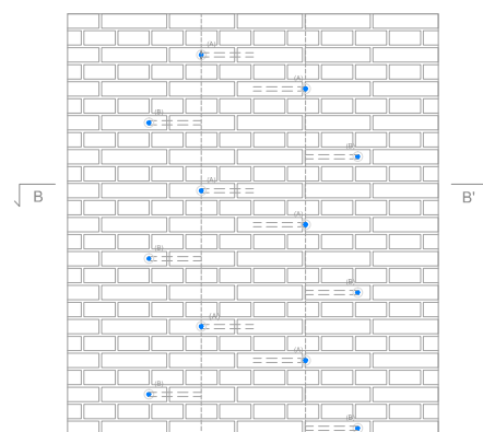
ELEVATION B
