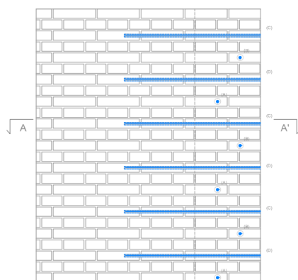
ELEVATION A
